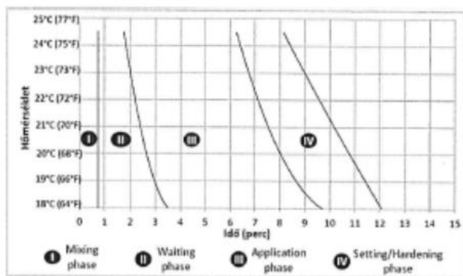
I. ábra A keverési, várakozási, alkalmazási és keményedési/keményedési idők grafikonja a szobahőmérséklet függvényében.
