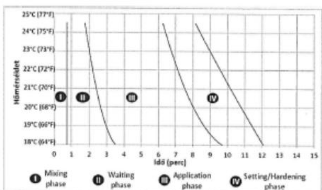
I. ábra A keverési, várakozási, alkalmazási és kikeményedési/kezdőkeményedési idők grafikonja a szobahőmérséklet függvényében.
