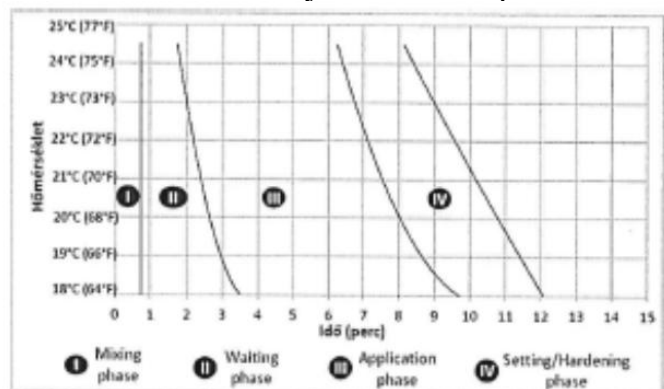
I. ábra A keverési, várakozási, alkalmazási és keményedési/keményedési idő grafikonja a szobahőmérséklet függvényében. A táblázatban feltüntetett idő 50 a 10% relatív páratartalom mellett végzett vizsgálatokból származik. Az időt idővel lehet csökkenteni, és a szobahőmérséklet és az alkalmazott keverési/keményedési rendszer függvényében hosszabbak, vagy rövidebbek lehetnek.
