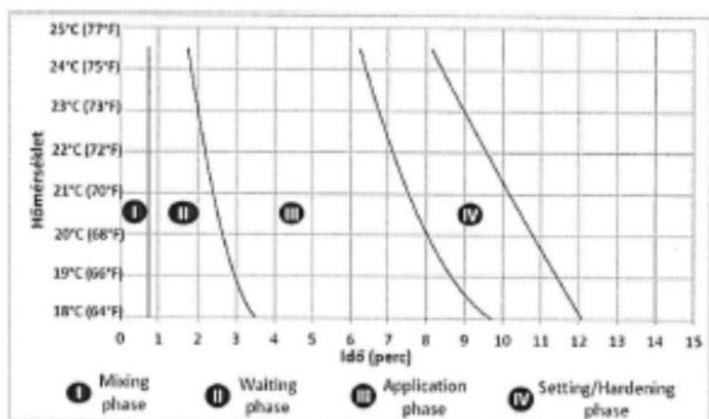
I. ábra A keverési, várakozási, alkalmazási és kikeményedési/harményedési idek grafikonja a szobahőmérséklet függvényében.
